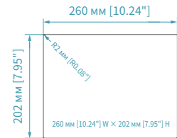
Размеры отверстия
