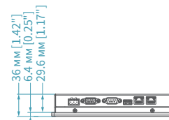
Вид снизу
