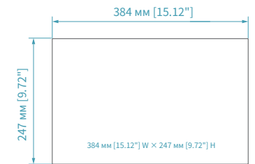
Размеры отверстия
