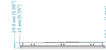
Вид снизу
