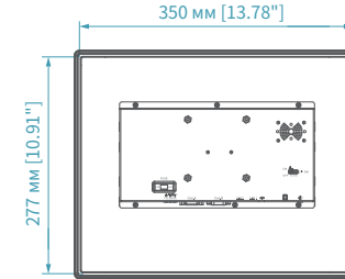
Вид сзади
