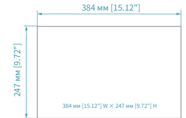
Размеры отверстия
