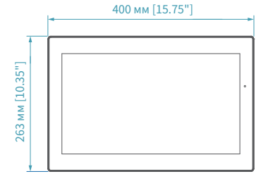
Вид спереди
