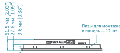
Вид снизу
