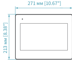
Вид спереди
