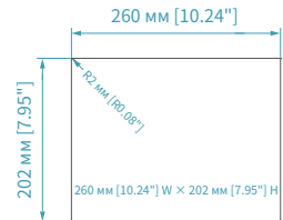
Размеры отверстия
