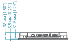
Вид снизу
