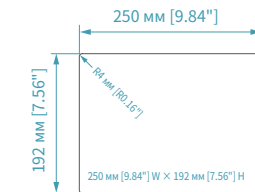
Размеры отверстия
