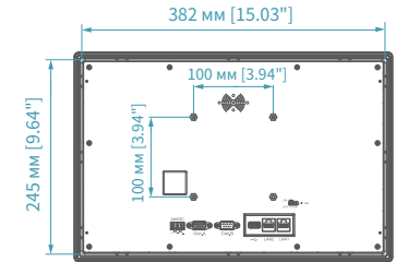
Вид сзади
