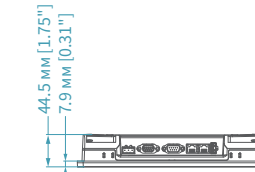
Вид снизу
