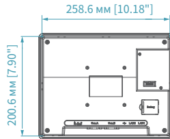
Вид сзади
